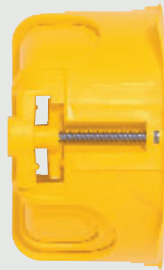
Cloison sèche avec de larges étriers rétractables
