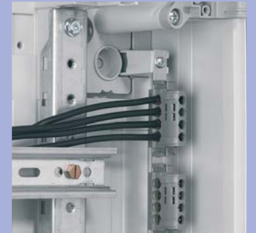
Bornier IP 2X montage vertical ou horizontal avec réf. 200 50
