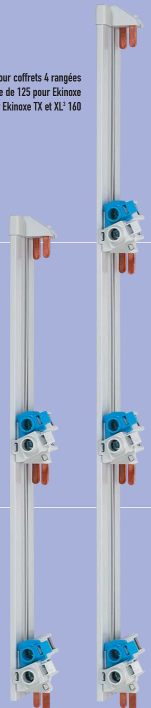
Peignes d'alimentation verticale 63 A
